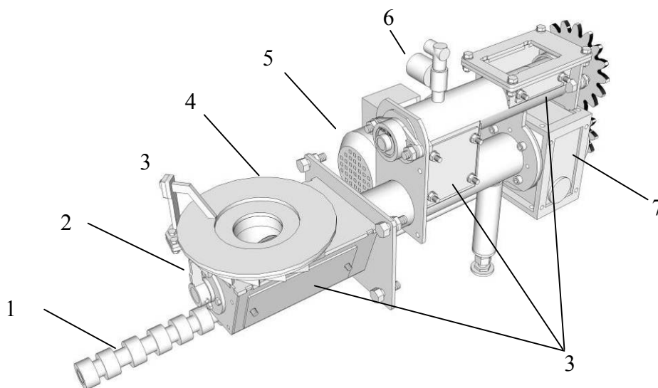
Рис. 8 - Устройство котла в разрезе
