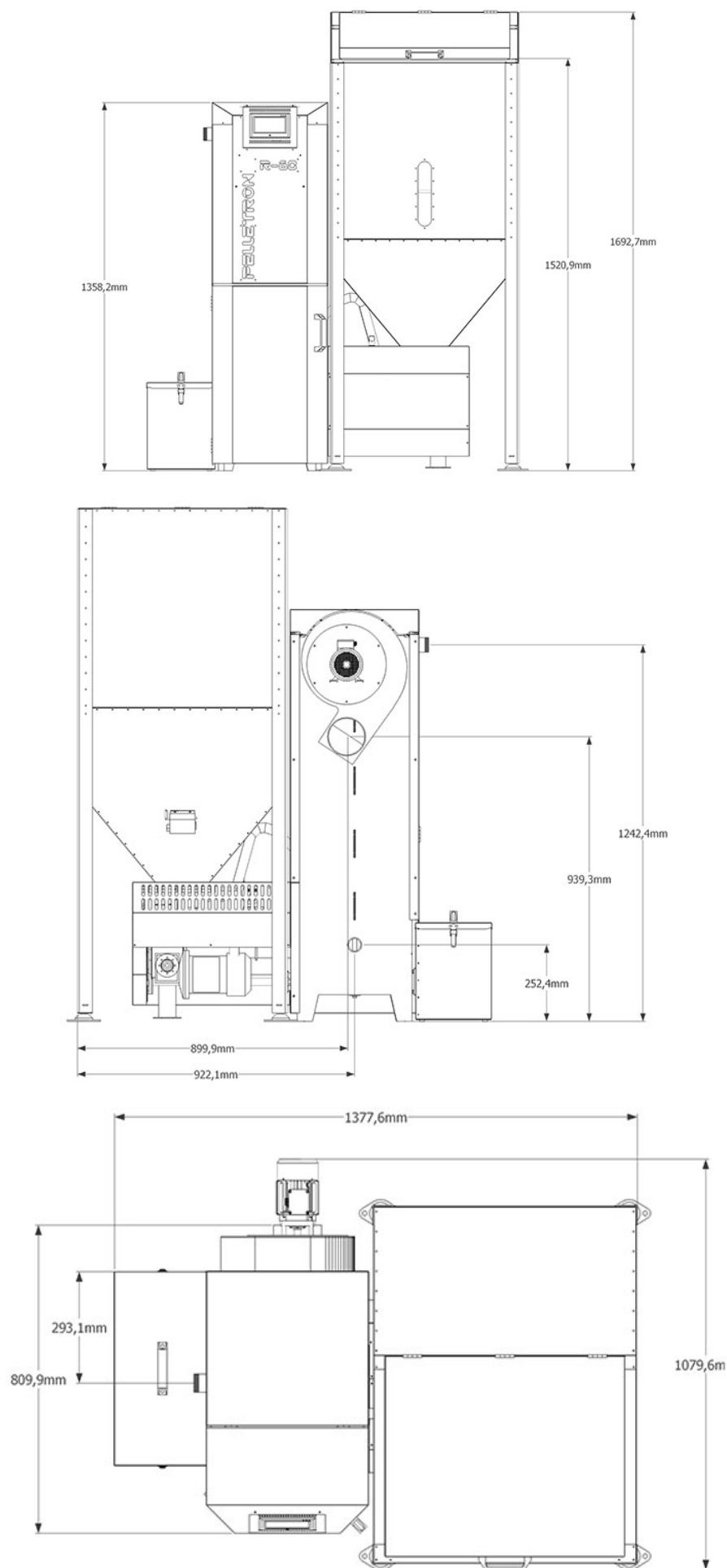
Рис. 2 - Габаритные размеры котла R60
