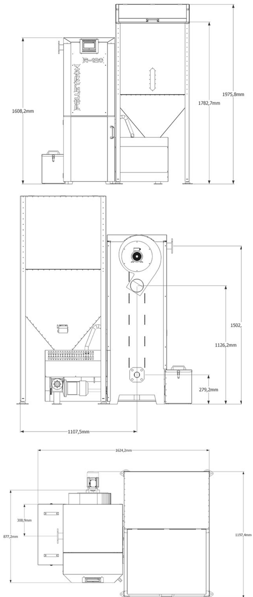
Рис. 3 - Габаритные размеры котла R120
