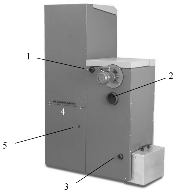
Рис. 4 - Общий вид котла R30
