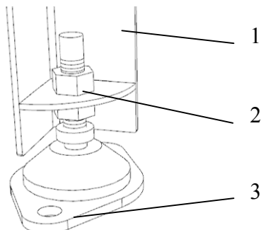
1 - ножка бункера, 2 - регулируемая опора, 3 - рамка опоры
