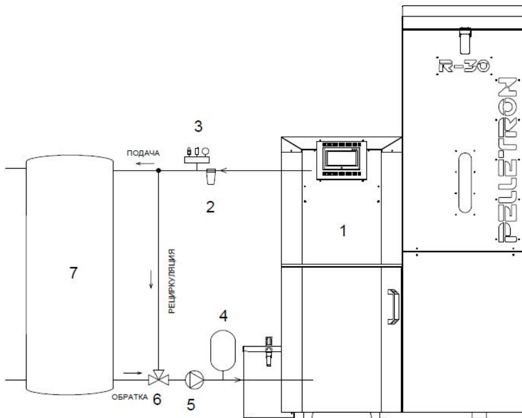
1 - котел, 2 - фильтр, 3 - предохранительный клапан и манометр, 4 - расширительный бак, 5 - насос рециркуляции, 6 - термостатический трехходовой клапан, 7 - буферная емкость
