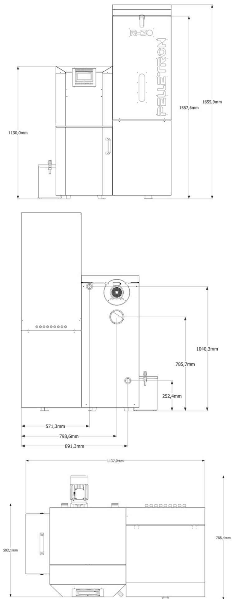
Рис. 1 - Габаритные размеры котла R30
