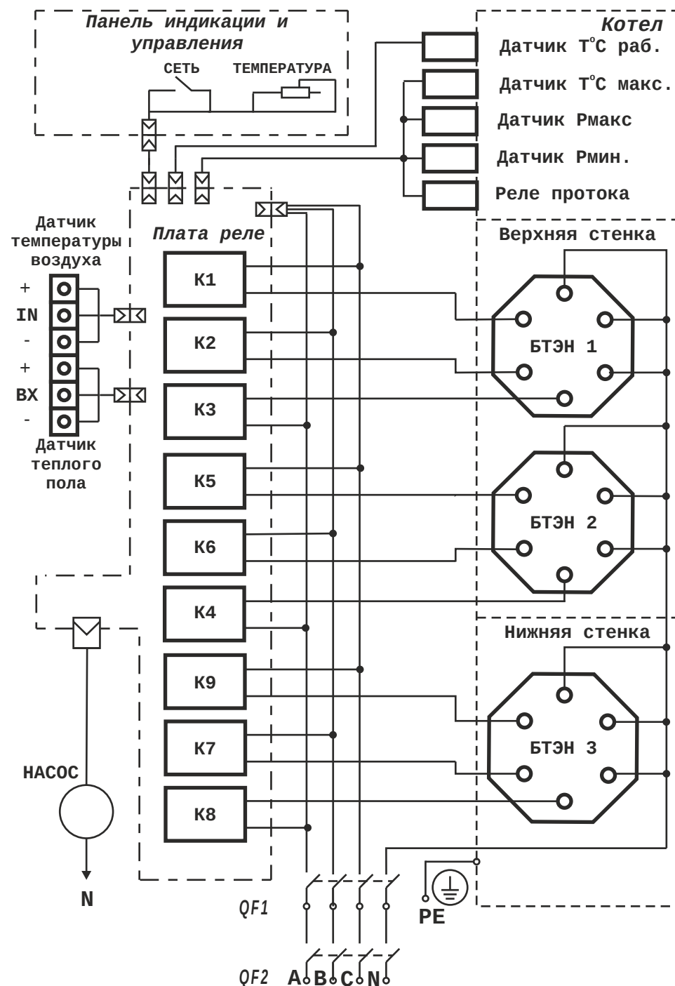
Рис. 5 Схема подключения
